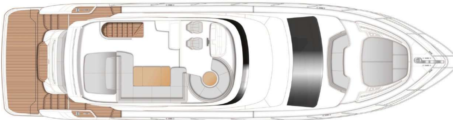
FLYBRIDGE
